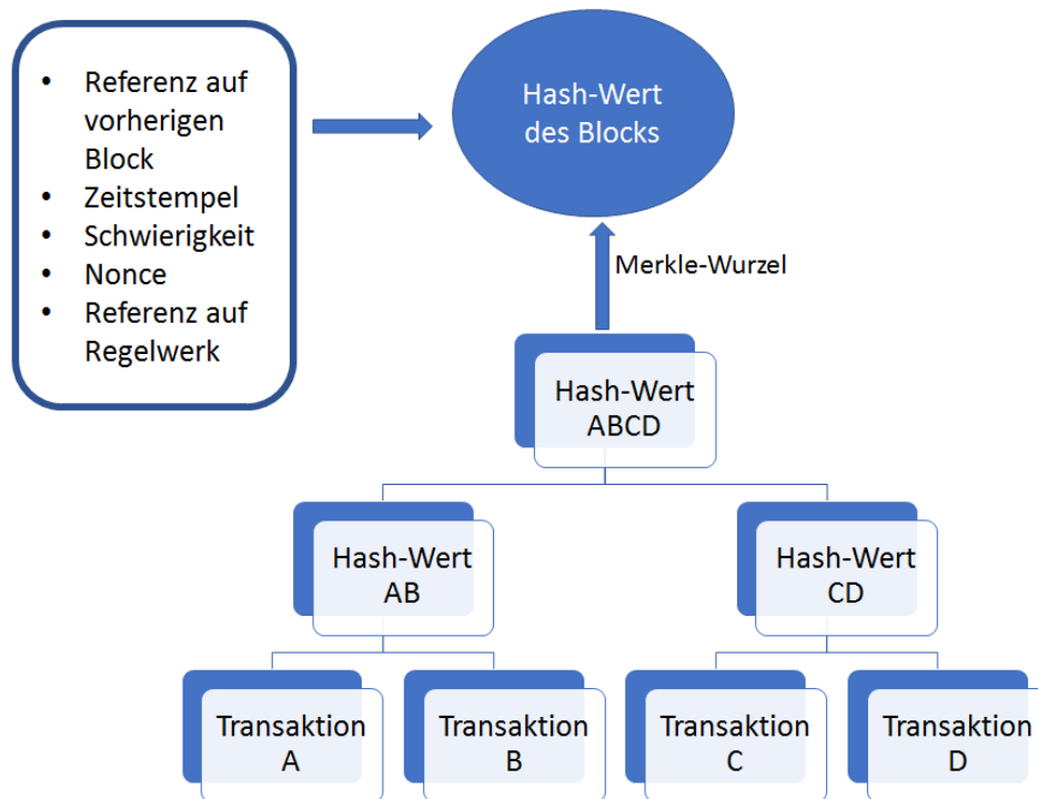
Abbildung 2: Aufbau eines Merkle-Baums und Erstellung eines Blocks 5
