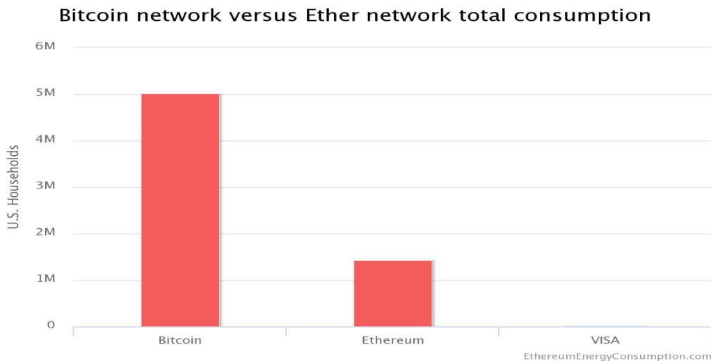
Abbildung 9: Gesamter Stromverbrauch des Bitcoin-, Ethereum- und VISA- Netzwerks pro Jahr in Relation zum Stromverbrauch eines durchschnittlichen US-Haushalts (der Betrieb von Banken wird bei der Untersuchung des VISA Netzwerks nicht berücksichtigt) 19
